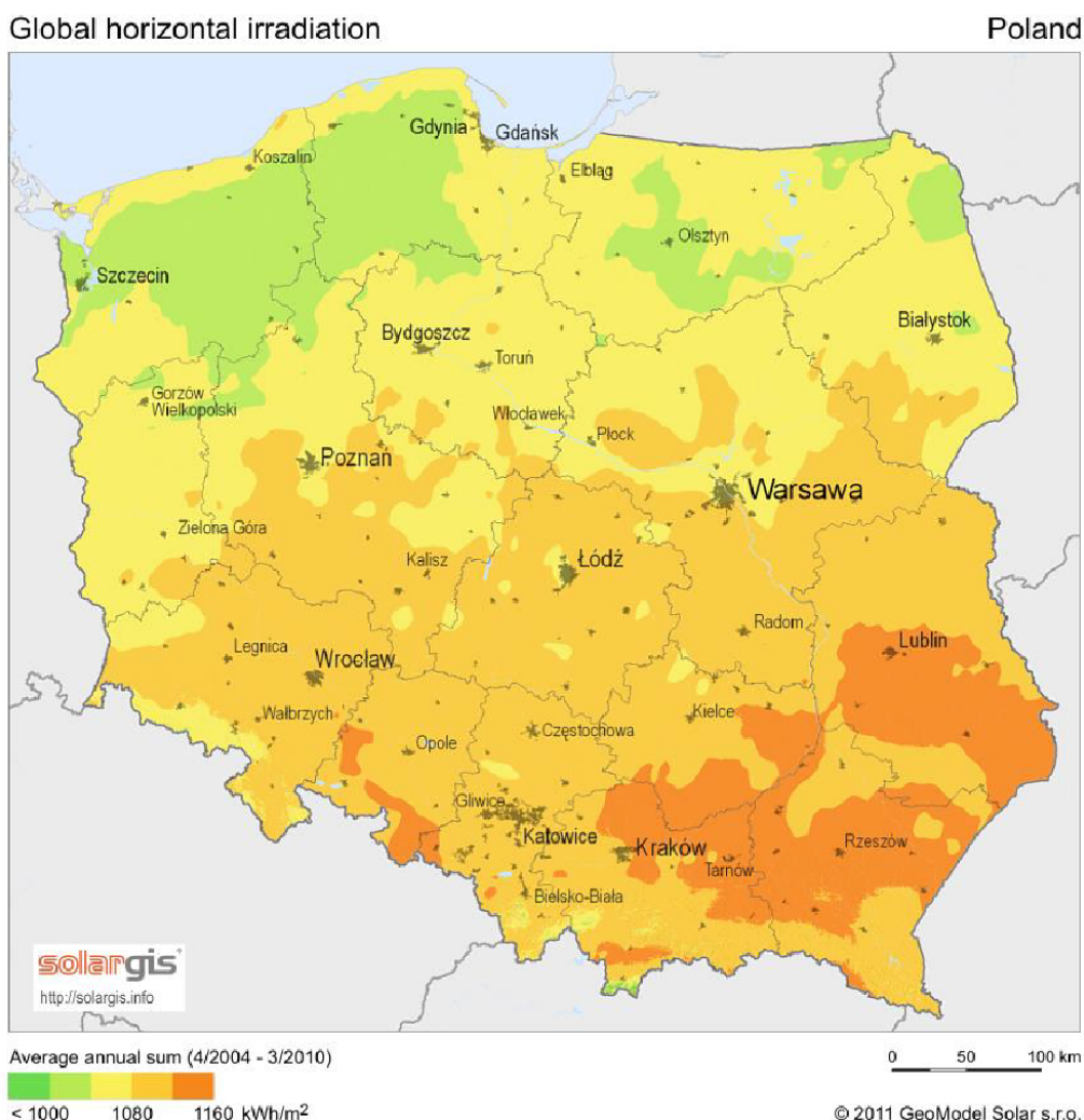
Rysunek 1 Rozkład promieniowania słonecznego na terenie Polski
